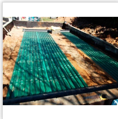
Gruntowy wymiennik ciepła GEOSTRONG – w fundamentach rozszelony
